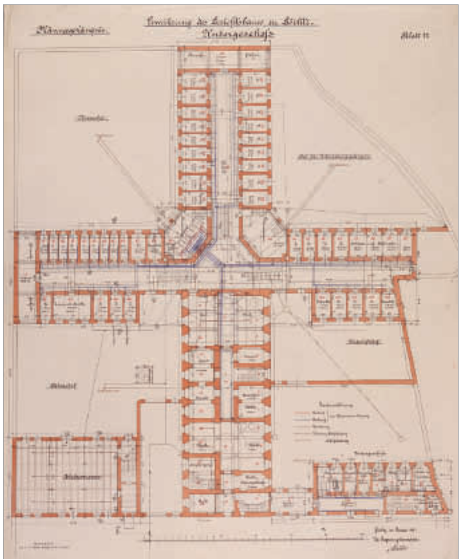
12 Grundriss des Görlitzer Gerichtsgefängnisses, Erdgeschoss, 1911
