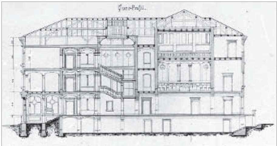
8 Schnitt durch das Gerichtshaus.
